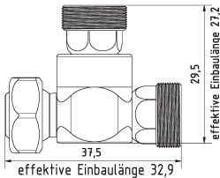
1-WV-R-2K T-Stück für Ring und Düse T-piece fo ring and nozzle
