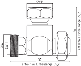
1-WV-R Verschlussstück zu Ringdüse locking tappet to ring nozzle
