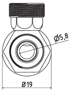
1-WI Winkelstück für Leitungen corner piece for pipelines
