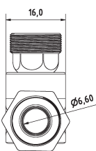
1-WV-R-2K T-Stück für Ring und Düse T-piece fo ring and nozzle
