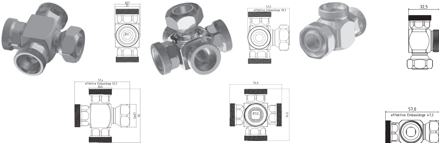
2-WV-3K Kreuz-Stück cross piece
