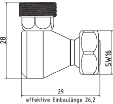
1-WI Winkelstück für Leitungen corner piece for pipelines
