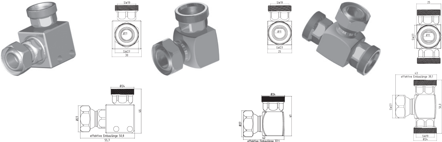
2-WI Winkelstück für Leitungen mit 2 Bohrungen corner piece for pipelines with 2 bore hole
